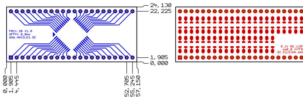
Bild 1. Obere Seite (Links) und untere Seite (rechts). Alle Abmessungen sind in Millimeters angegeben.
